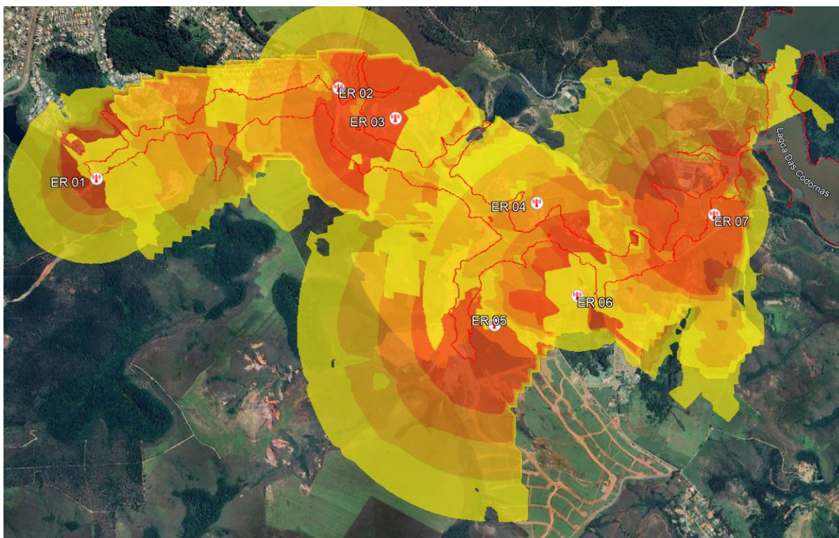
Figura 3: Cobertura sonora maior que 70Db do sistema de alerta de Lagoa Grande.
