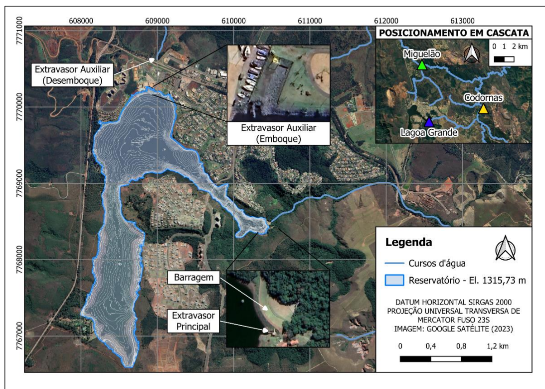
Figura 2: Visualização em planta do arranjo da barragem Lagoa Grande
